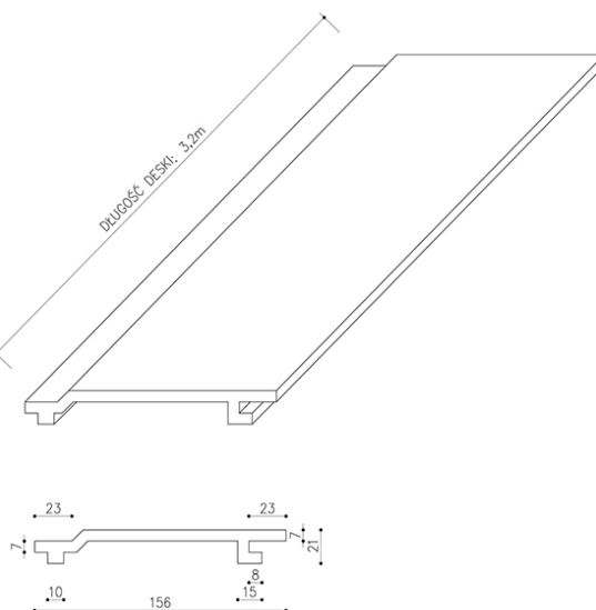
DESKA ELEWACYJNA PREMIUM II GENERACJI 3200mm x 156mm x 21mm
